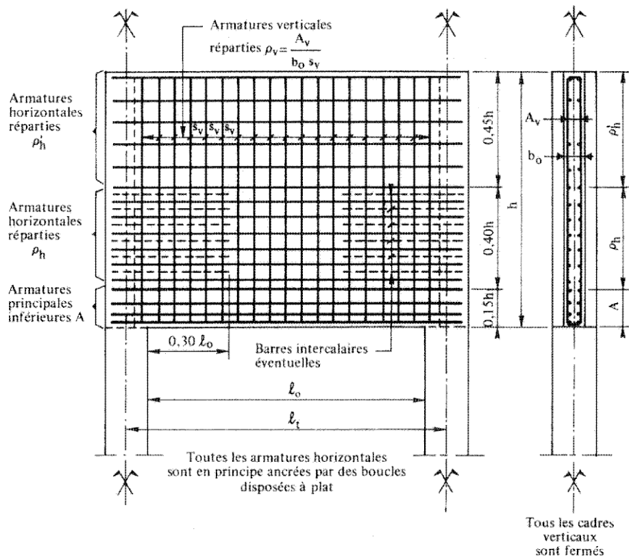
Figure 5 paroi fléchie à une travée h < l_t ( l_t = \min(l_o; 1, 15 l_o) )
